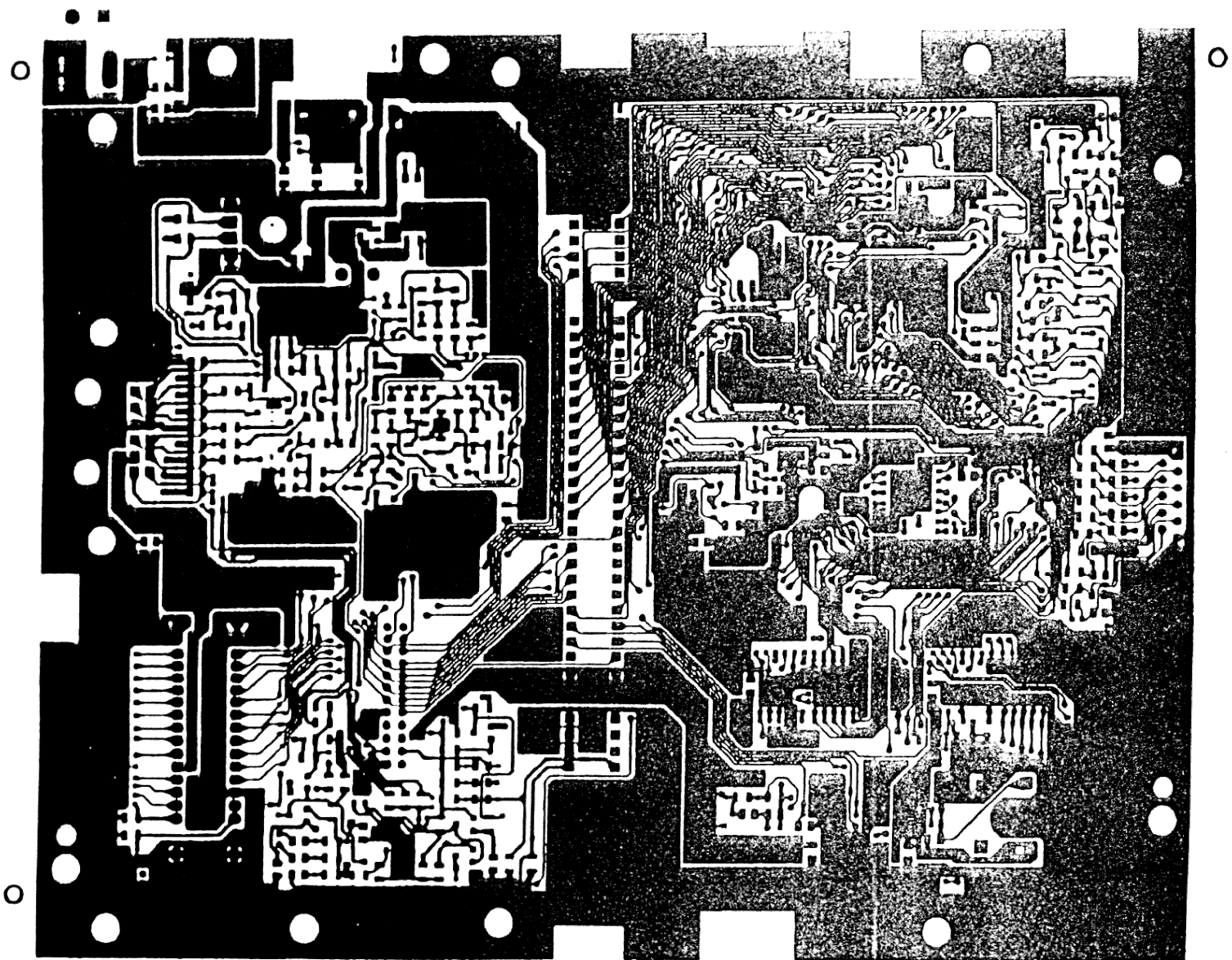
LAYOUT DE TRILHAS (DISCRETOS)
