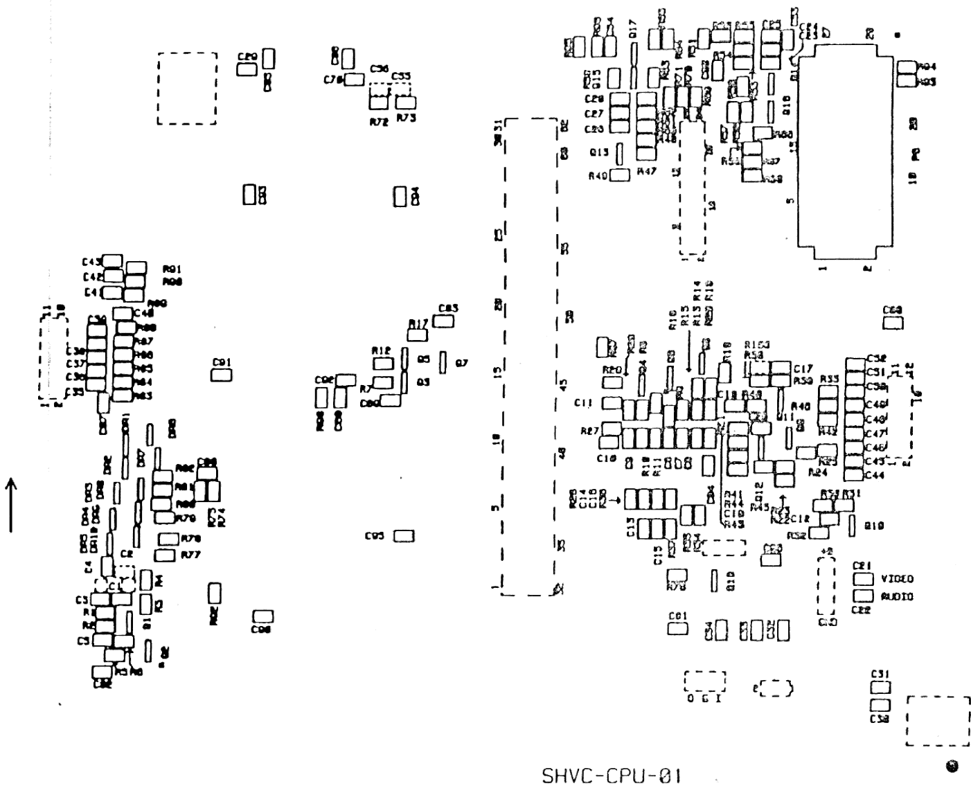
LAYOUT DE COMPONENTES (DISCRETOS)
