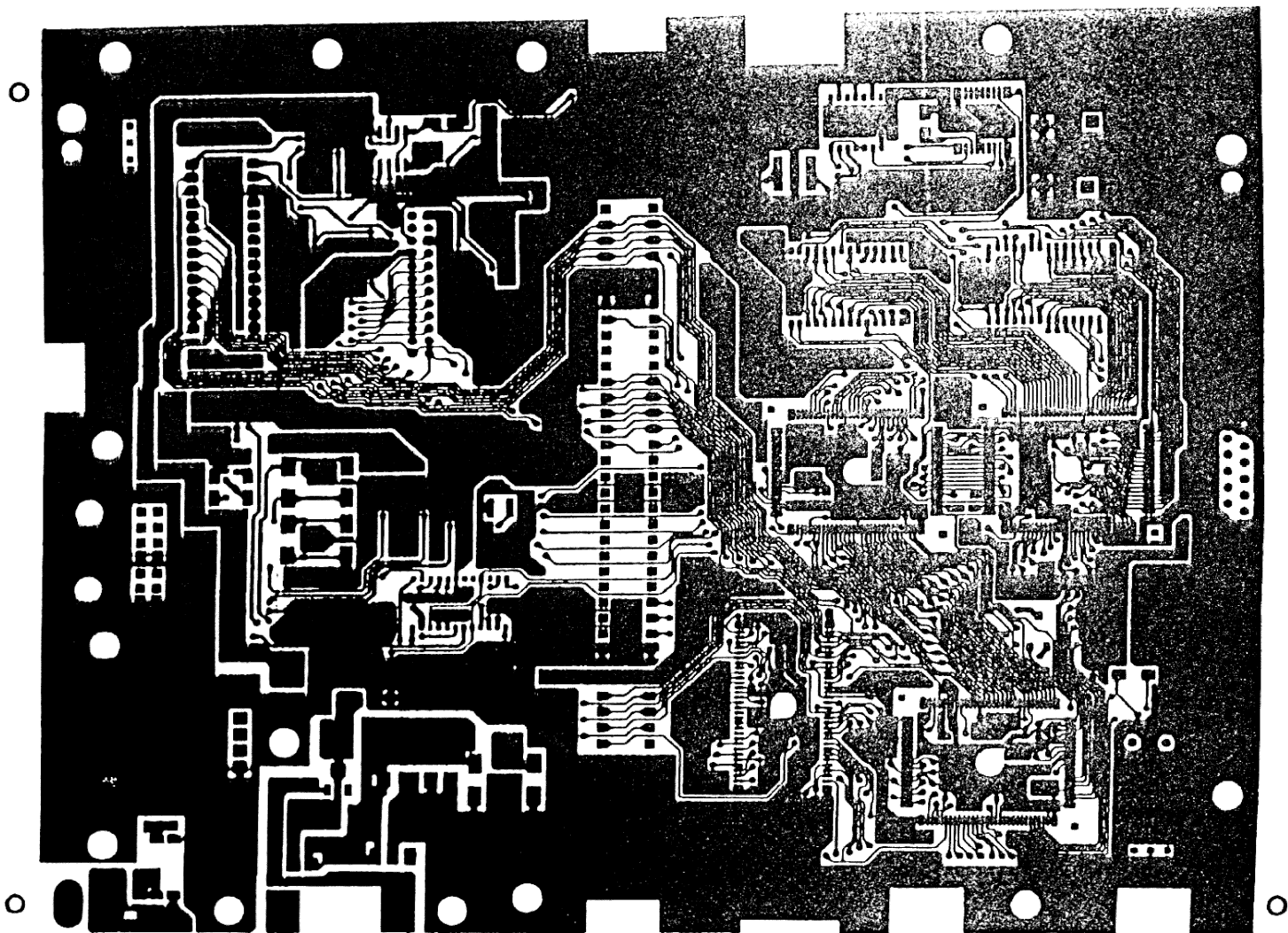
LAYOUT DE TRILHAS (CI)
