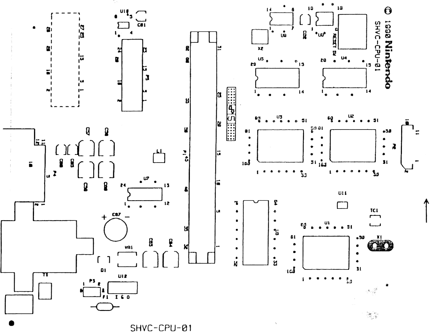
LAYOUT DOS COMPONENTES (CI)
